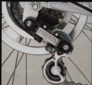
Simplex rear derailleur
